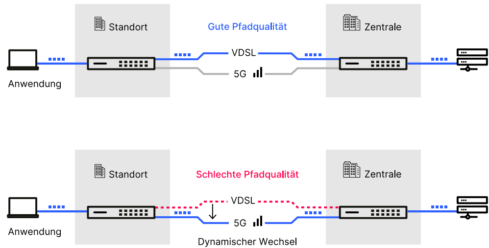
Abbildung 2: Funktionales Prinzip von Dynamic Path Selection
