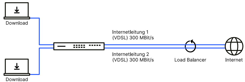
Abbildung 1: Active / Active-Verbund bzw. Load Balancing
