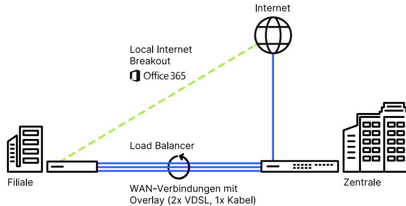
Abbildung 3: SD-WAN-Szenario mit Load Balancing, Local Internet Breakout und Dynamic Path Selection
